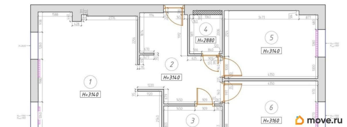
ПЛАН ОБМЕРНЫЙ
