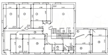
План 2-го этажа здания по адресу: г. Альметьевск, ул. Индустриальная, д. 23 В
