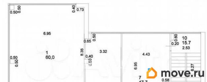
План 2 этажа
