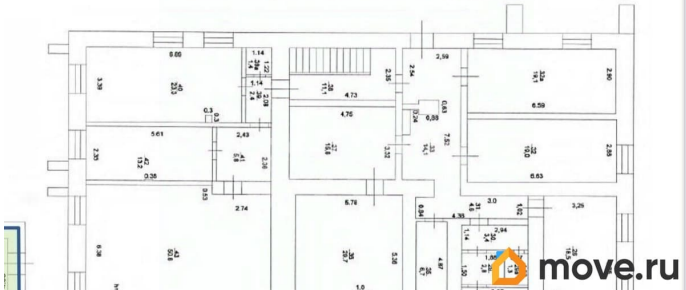
План 1 этажа (помещения 2Н площадью 242,3 кв. м.)
