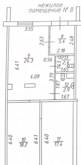
ПЛАН 1 ЭТАЖА НЕЖИЛОГО ПОМЕЩЕНИЯ №8
