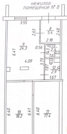
ПЛАН 1 ЭТАЖА НЕЖИЛОГО ПОМЕЩЕНИЯ №8
